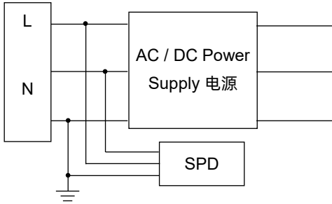
并联（一端口）
