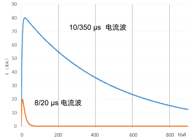
标准雷电测试波形
